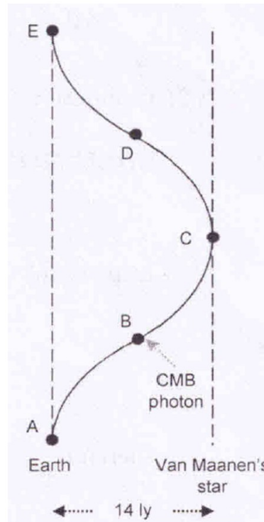
Figuur 1: Ruimtetijsdiagram voor de schematische weergave van de Tweelingparadox.
