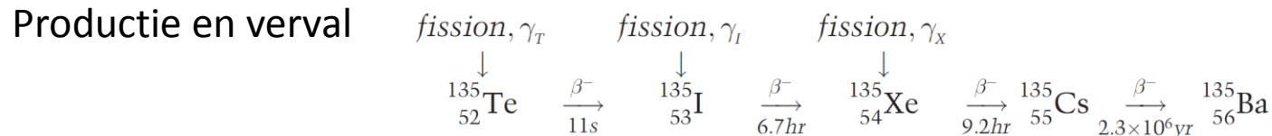
Thermal Fission Product Yields in Atoms per Fission
