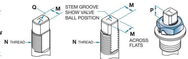
STEM DIMENSIONS DD
