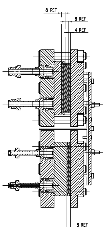
SECTION A-A
