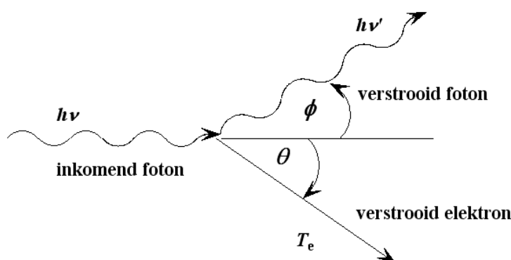
Figuur 2: Compton verstrooiing van een foton aan een elektron kan worden beschouwd als een elastische botsing.
