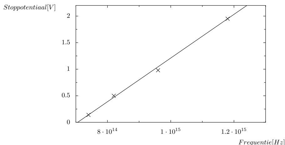
Figuur 1: Fotoelektrisch effect: de stoppotentiala is uitgezet als functie van de frequentie van het invallende licht.
