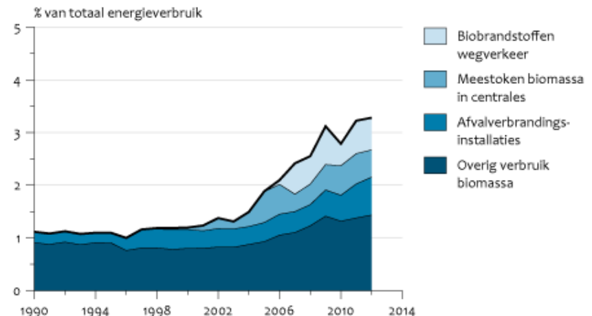
Eindverbruik biomassa
