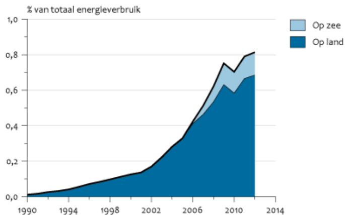
Eindverbruik windenergie
