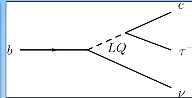
Leptoquark
