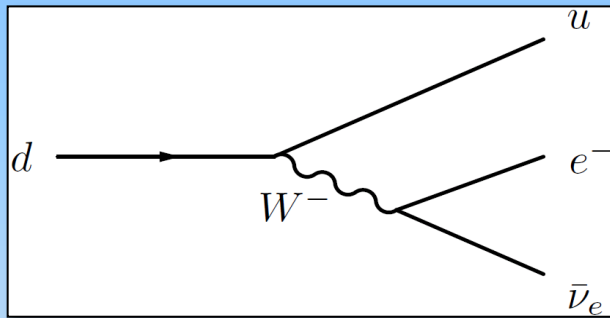
SM
